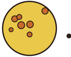
Io
