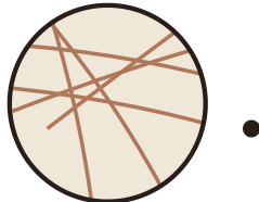
Europa
