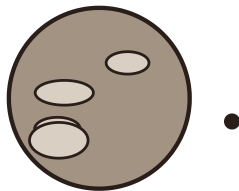
Ganymede
