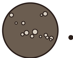
Callisto
